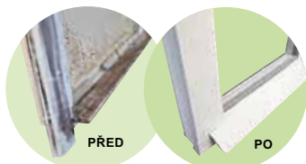
VÝMĚNA SKLA V DŘEVĚNÉM OKNĚ
